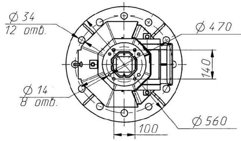
Вид сверху (1:10)
